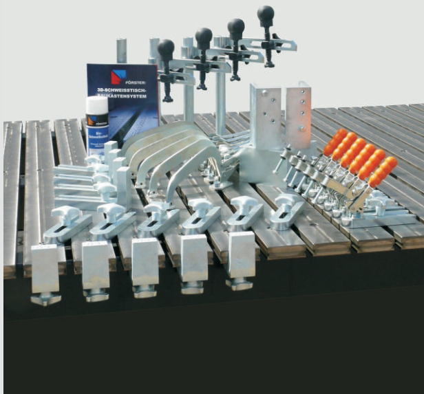
Комплект зажимов №2 для сваривания труб
