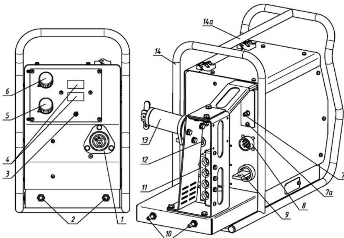
Внешний вид подающего механизма с установленной защитной рамой
