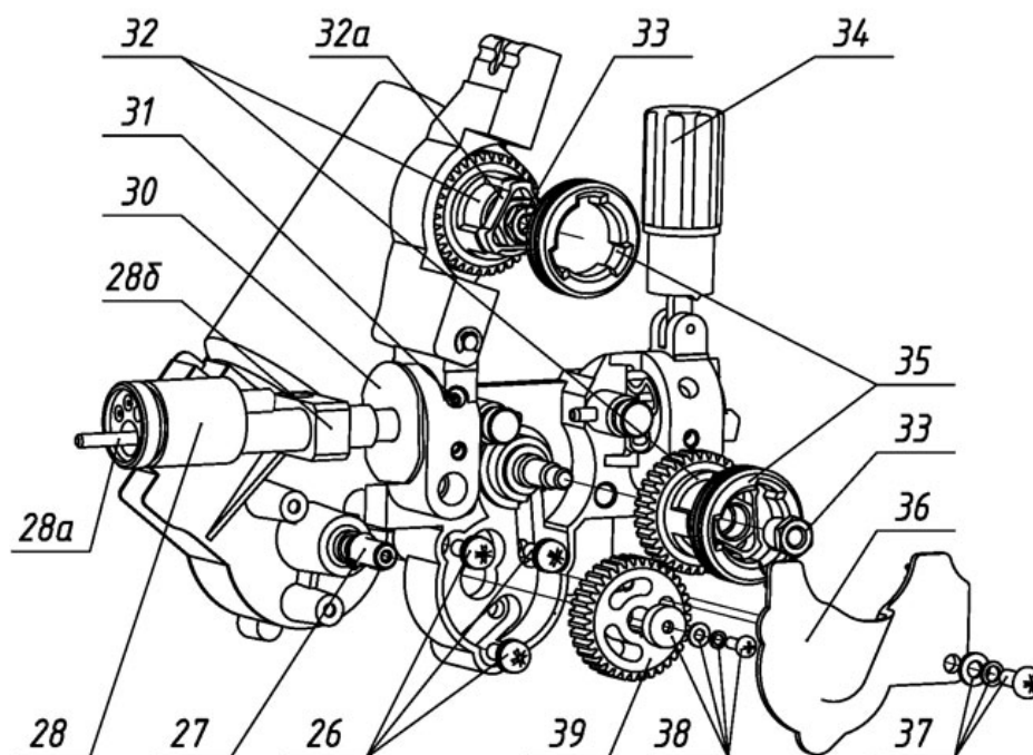
Механизм подачи проволоки SSJ-21 с евроразъемом
