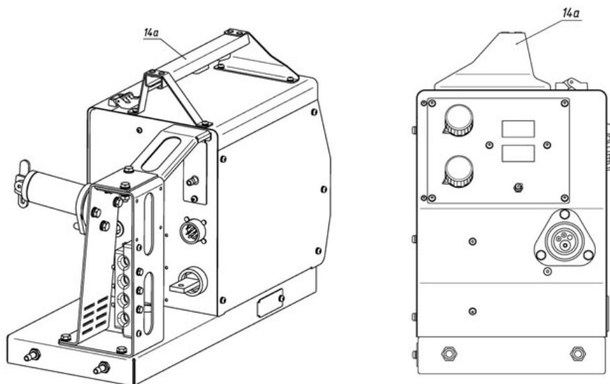
Внешний вид подающего механизма без металлической защитной рамы
